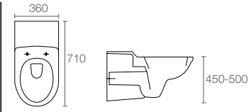
ODELA™ | K-1028D-00
