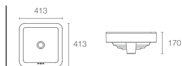
FOREFRONT™ | K-2661IN-0
