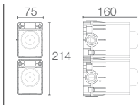
BEITOU™ K-99870T-CP
