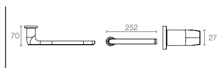
AVID™ | K-97498T-CP
