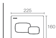
PEBBLE™ | K-5413IN-M-CP
