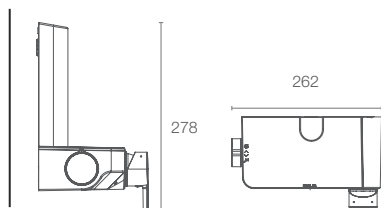
TOOBI™ K-75457IN-4-CP
