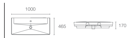
REVE™ | K-5026K-00
