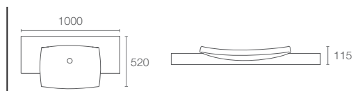
ESCALE™ | K-19034W-00
