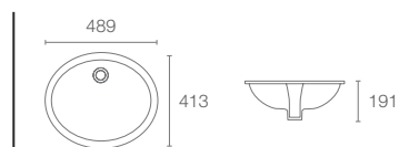
CAXTON™ | K-2210IN-0
