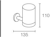
STILLNESS® | K-14463T-RGD
